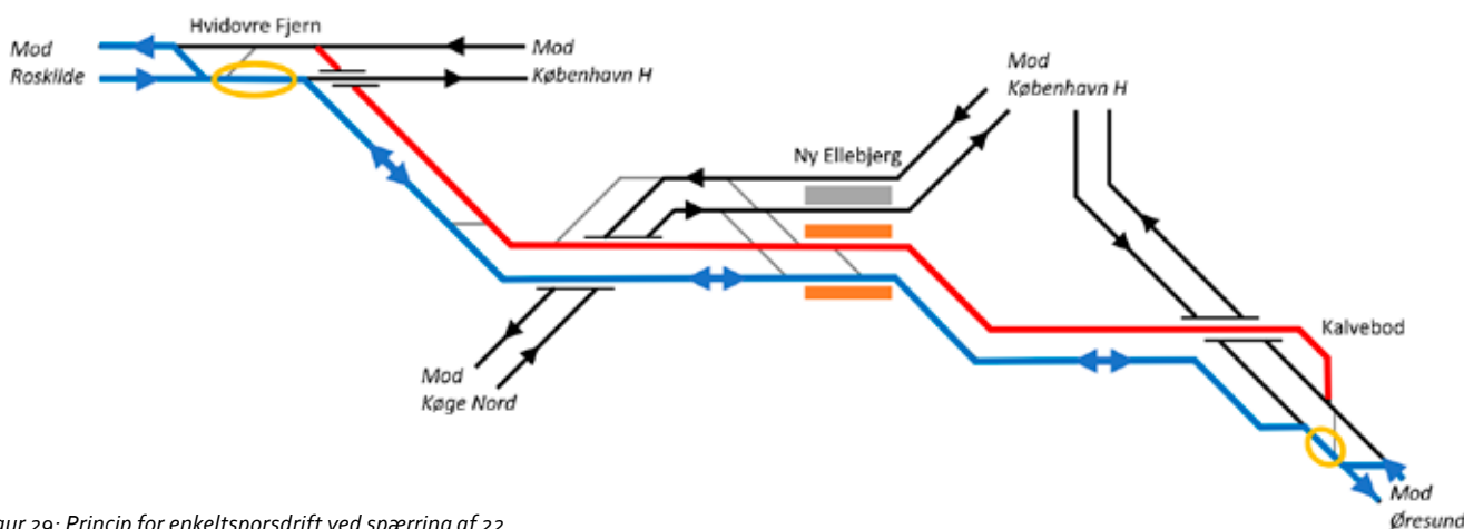
Figur 29: Princip for enkeltsporsdrift ved spærring af 22
