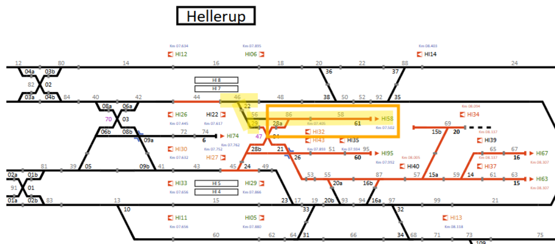
Sporspærring 20252013 og fejlretningssporspærring til manuel nulstilling af akseltællerafsnit TVS_HI47
