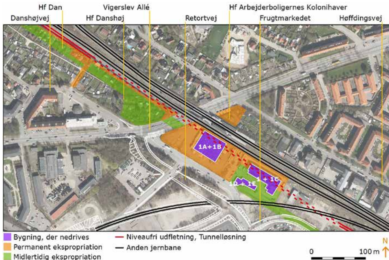
Figur 9 Oversigtskort over tunnelloøsningens arealbehov omkring Vigerslev Allé.
