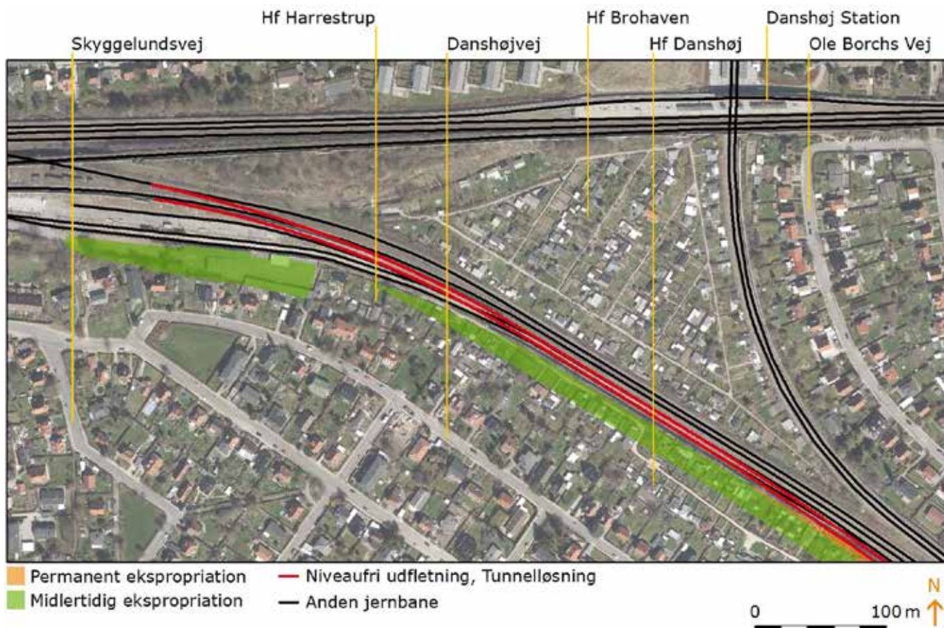
Figur 10 Oversigtskort over tunnelloøsningens arealbehov vest for Vigerslev Allé.
