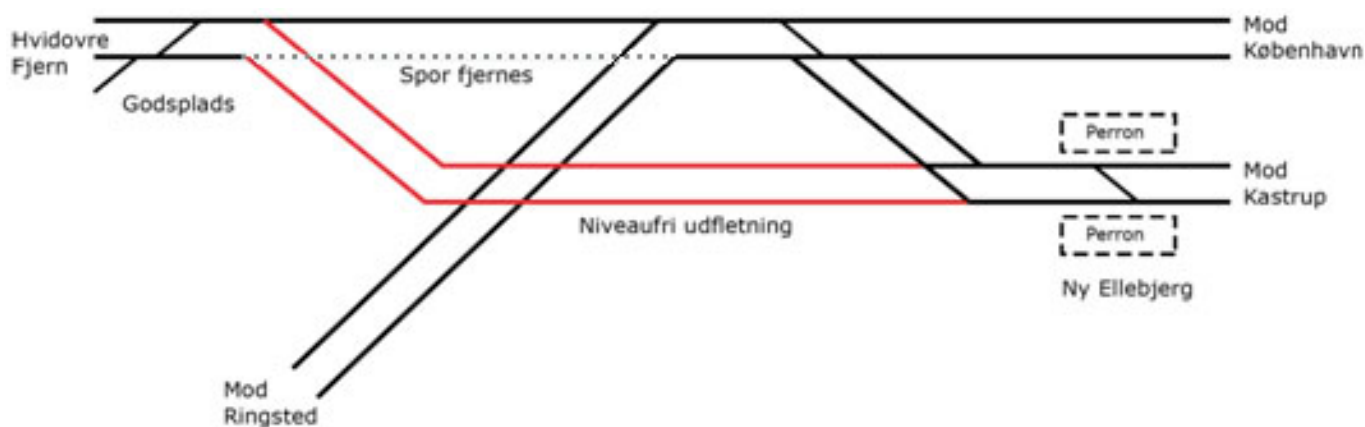
Figur 4 Sporplan for projektet
