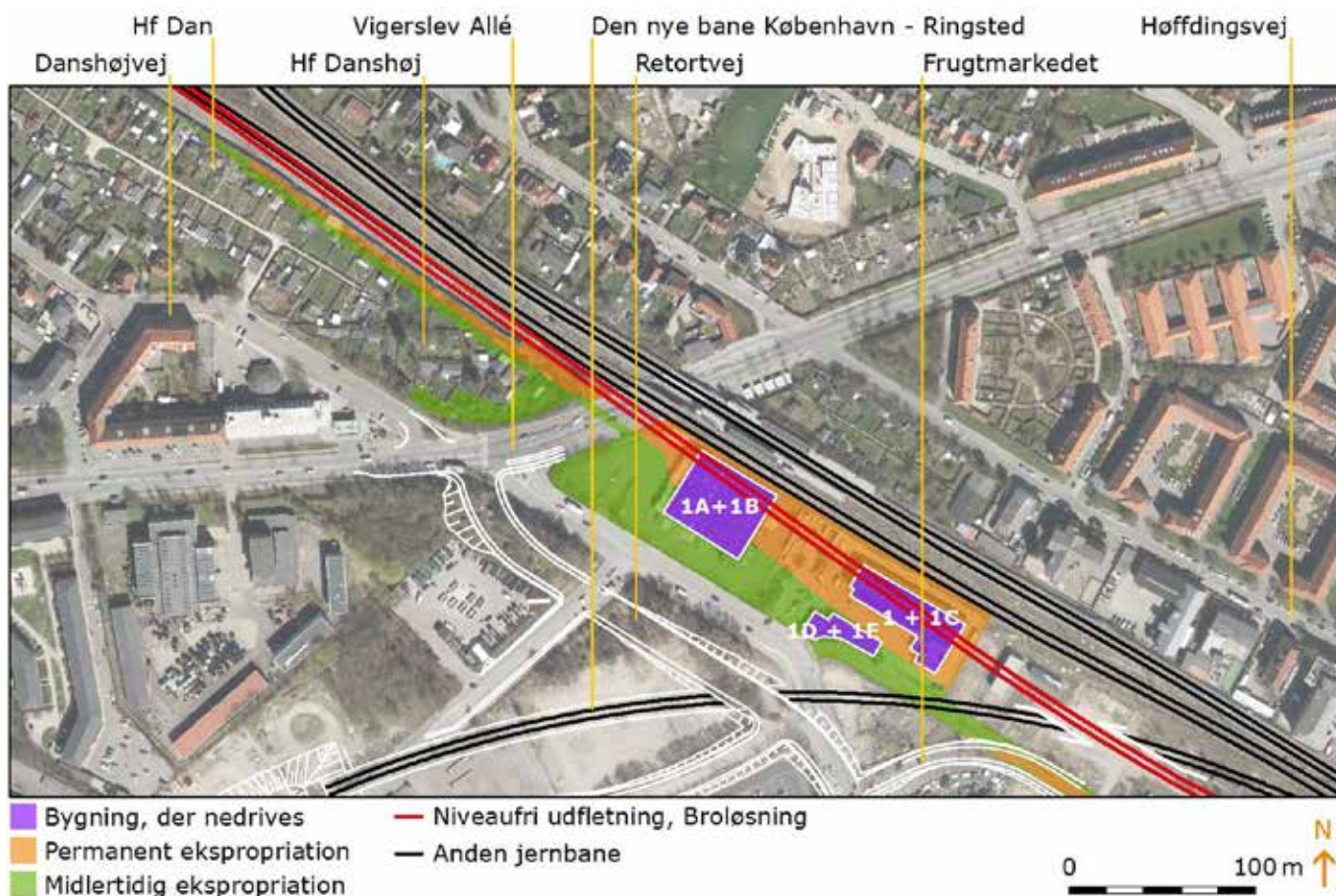
Figur 6 Oversigtskort over broløsningens arealbehov omkring Vigerslev Allé.
