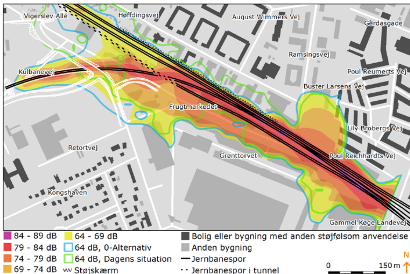
Figur 24 Oversigtskort over støjbilledet i tunnelens driftsfase.
