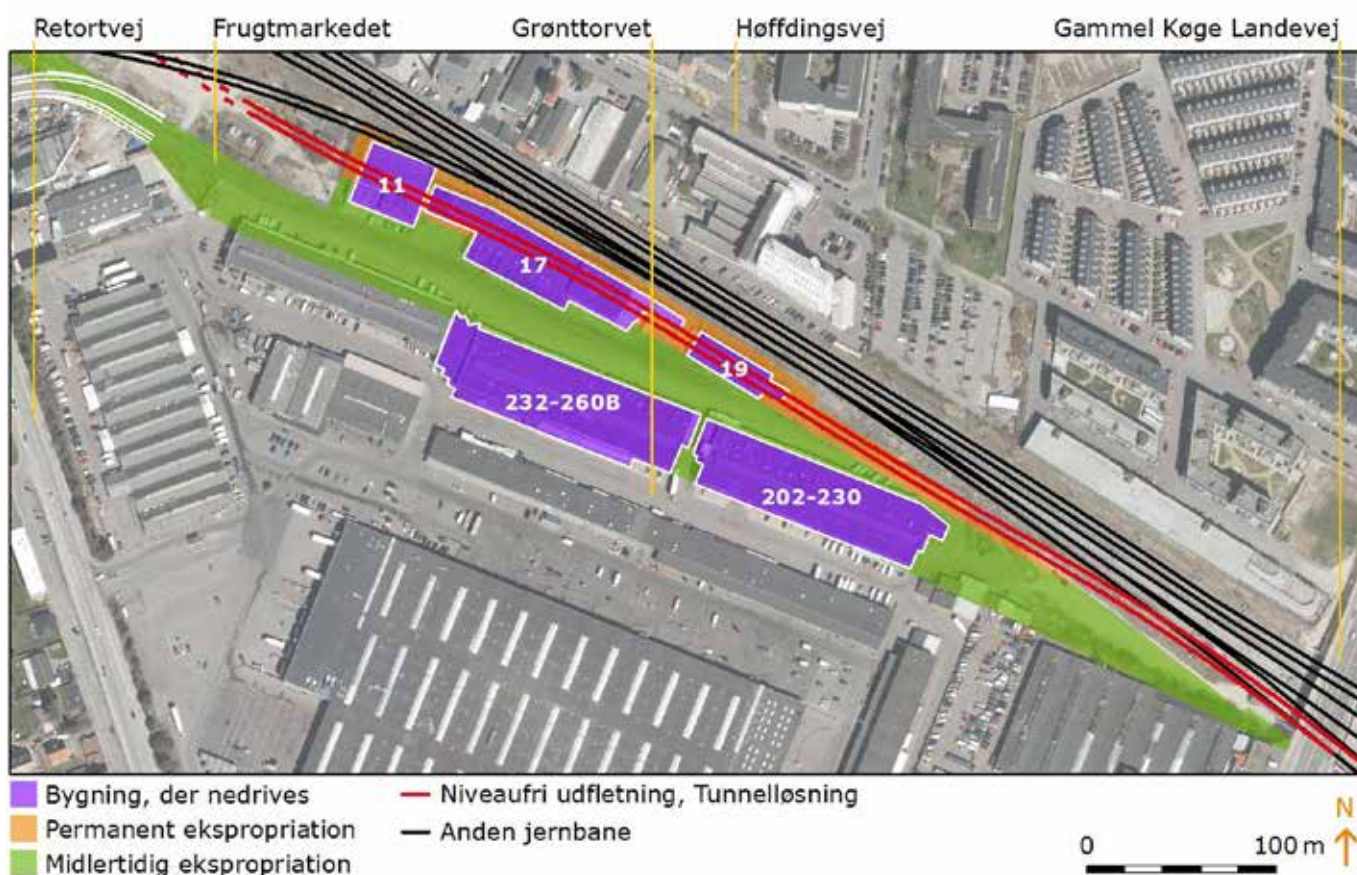
Figur 7 Oversigtskort over tunnelløsningens arealbehov ved grønttorvsområdet
