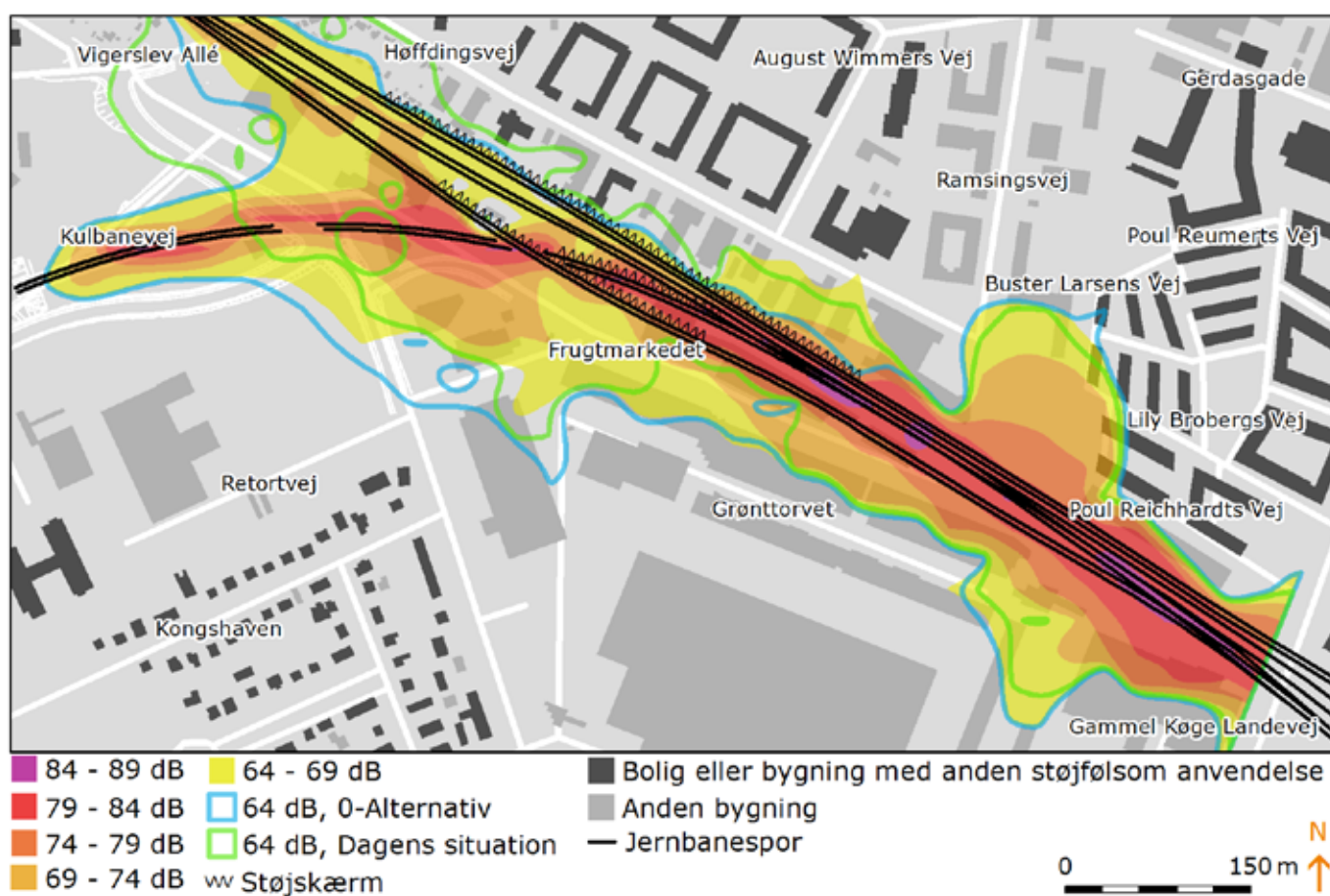
Figur 25 Oversigtskort over støjbilledet i broens driftsfase hvis den alternative støjskærm opføres.
