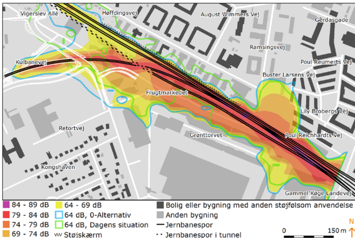
Figur 24 Oversigtskort over støjbilledet i tunnelløsningens driftsfase.
