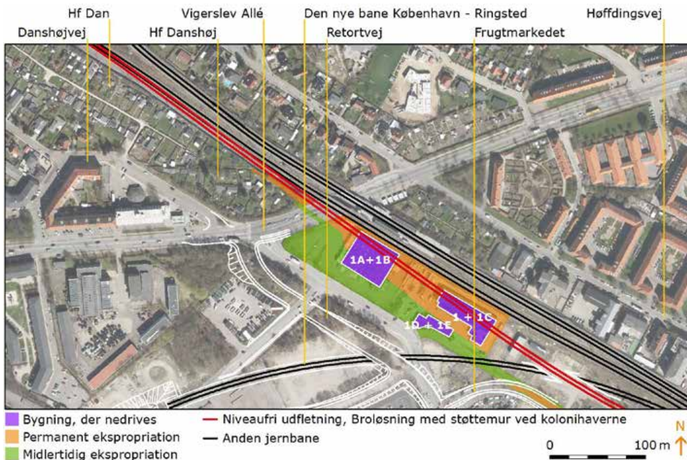
Figur 8 Oversigtskort over broløsningens arealbehov omkring Vigerslev Allé, hvis den alternative spunsløsning vælges.
