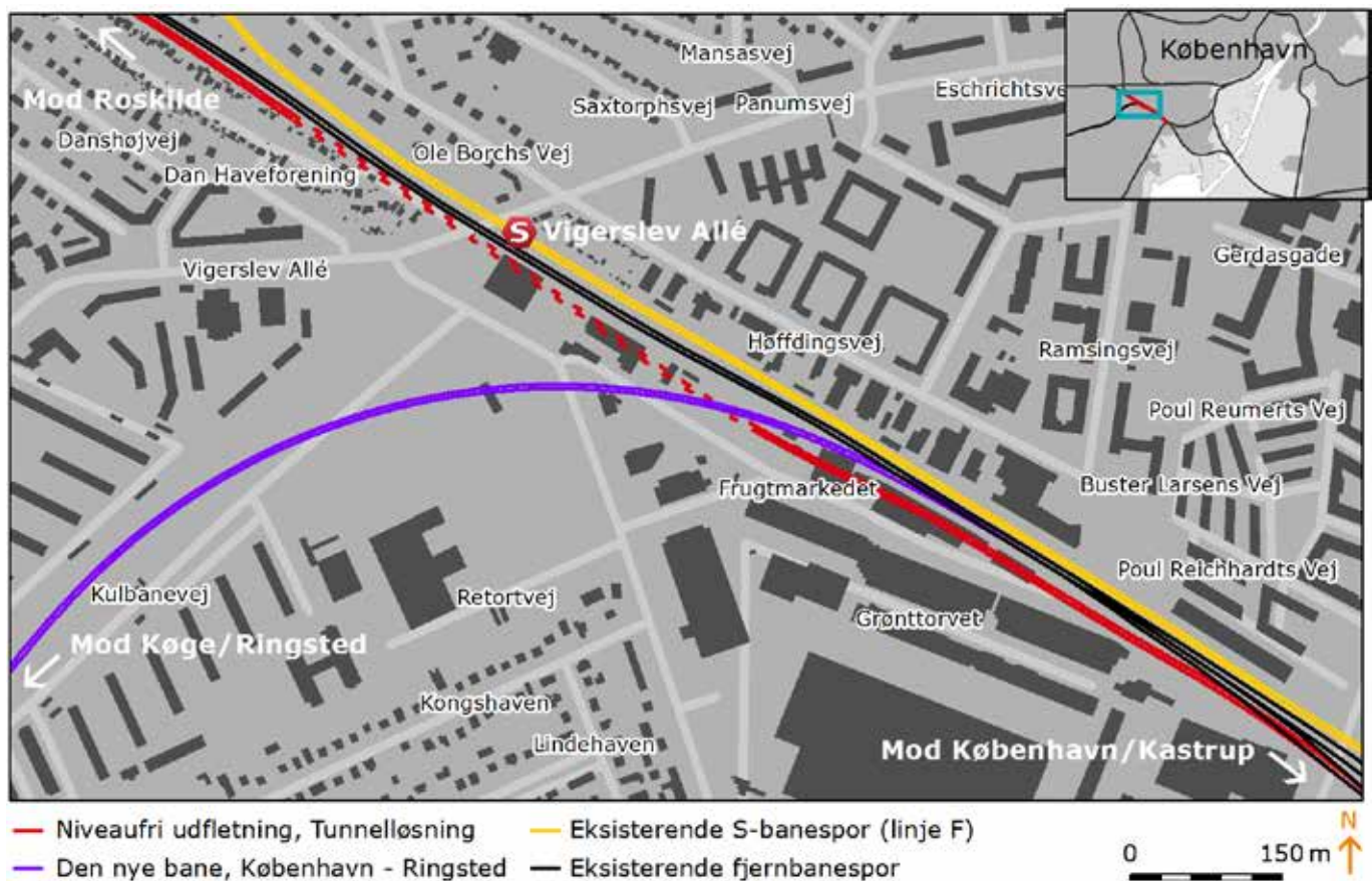
Figur 3 Oversigtskort over tunnelloseringen.
