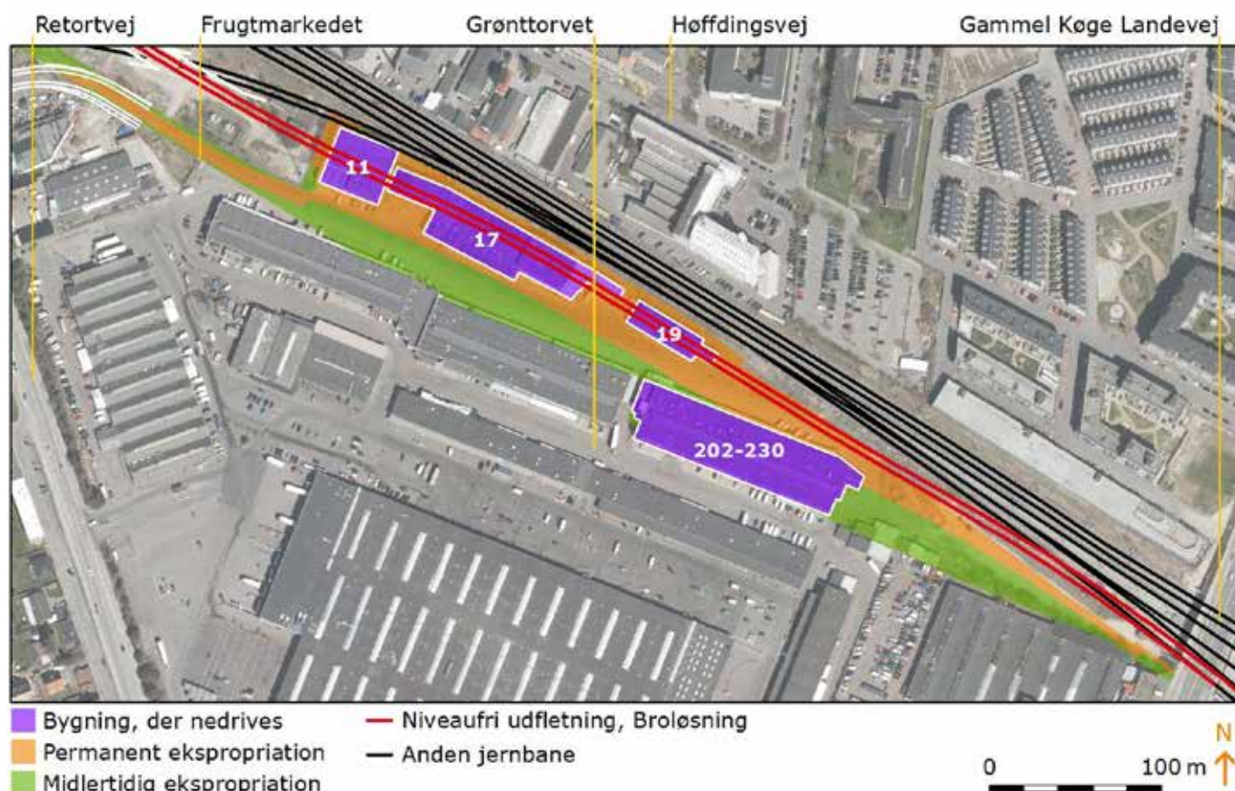
Figur 5 Oversigtskort over brøsløsnings arealbehov ved grønttorvsområdet.
