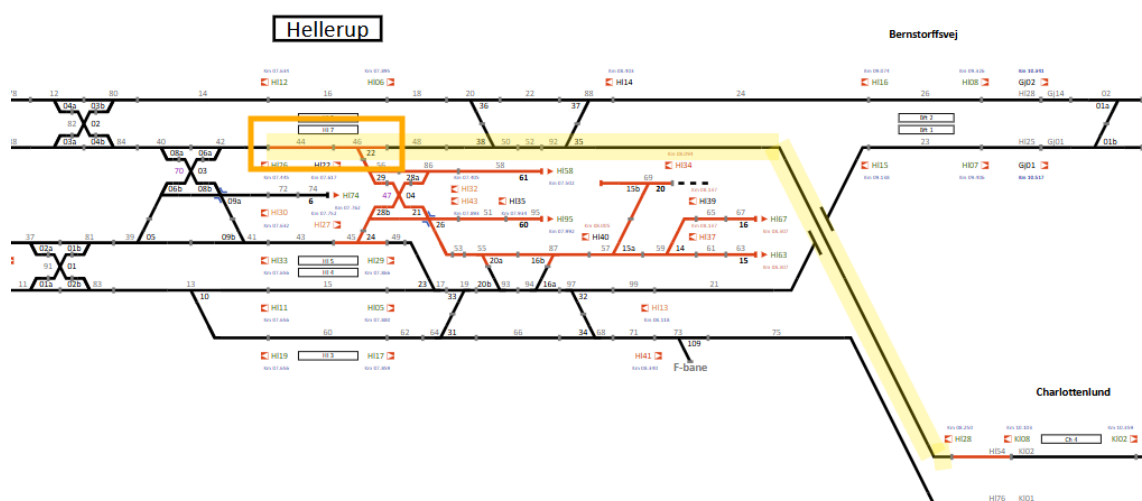
Sporspærring 20252632 og 20252825
