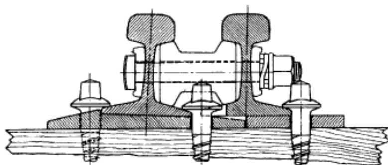
Figur 14. Tvangskinneprofil af almindeligt skinneprofil.
