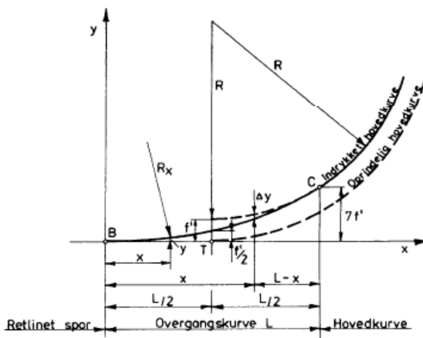
Figur 4. Overgangskurve mellem ret linie og cirkelbue udtrykt ved 4. gradsparabel.
