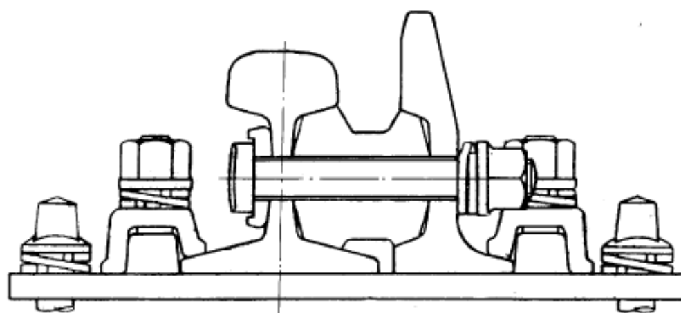
Figur 15. Højt tvangskinneprofil.
