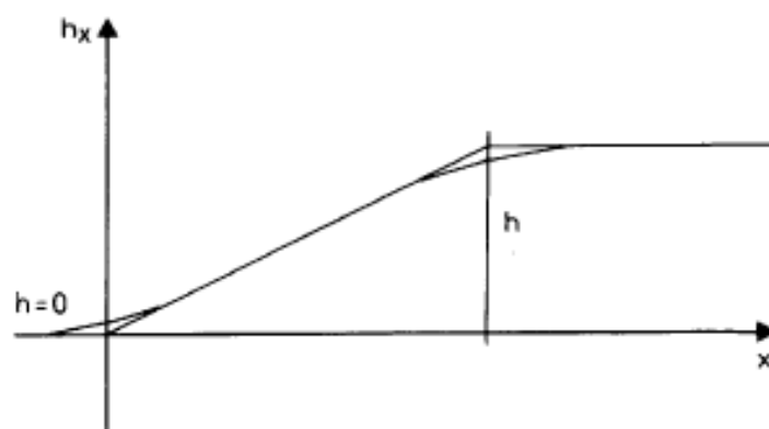
Figur 12. Retlinet overhøjderampe mellem ret spor og kurve
